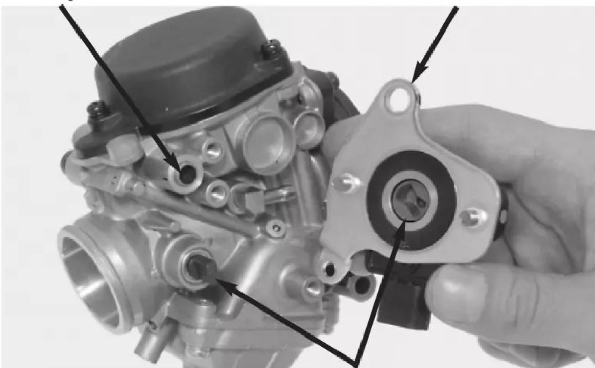
CARBURADOR Nº 1
