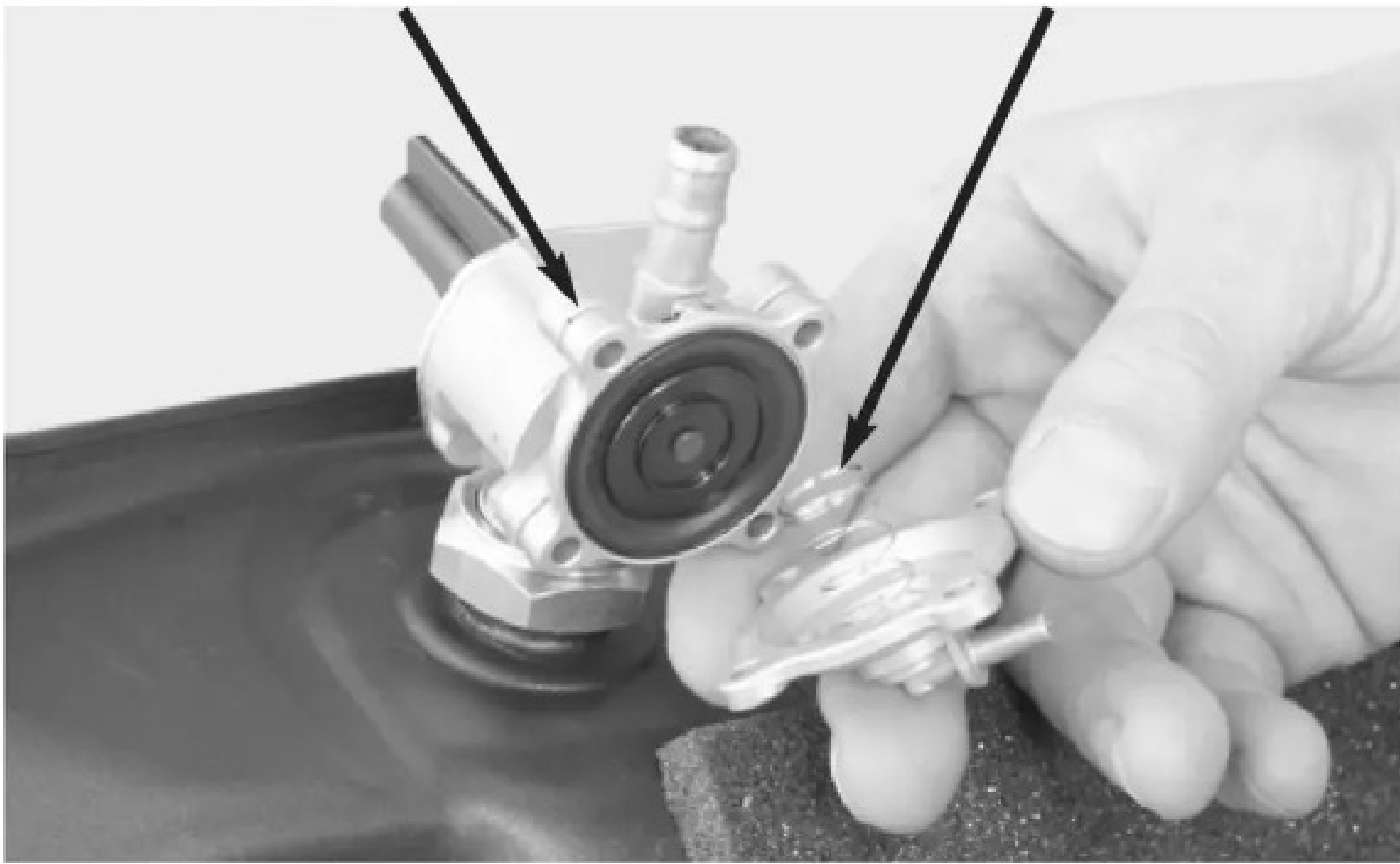
DIAFRAGMA/ESPAÇADOR MOLA
