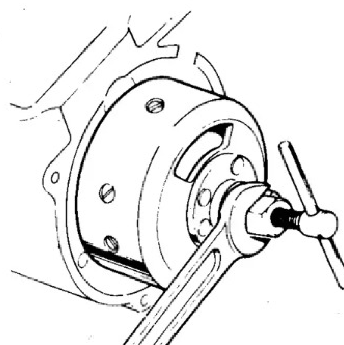
EXTRATOR DO ROTOR N.º 07933-0010000
