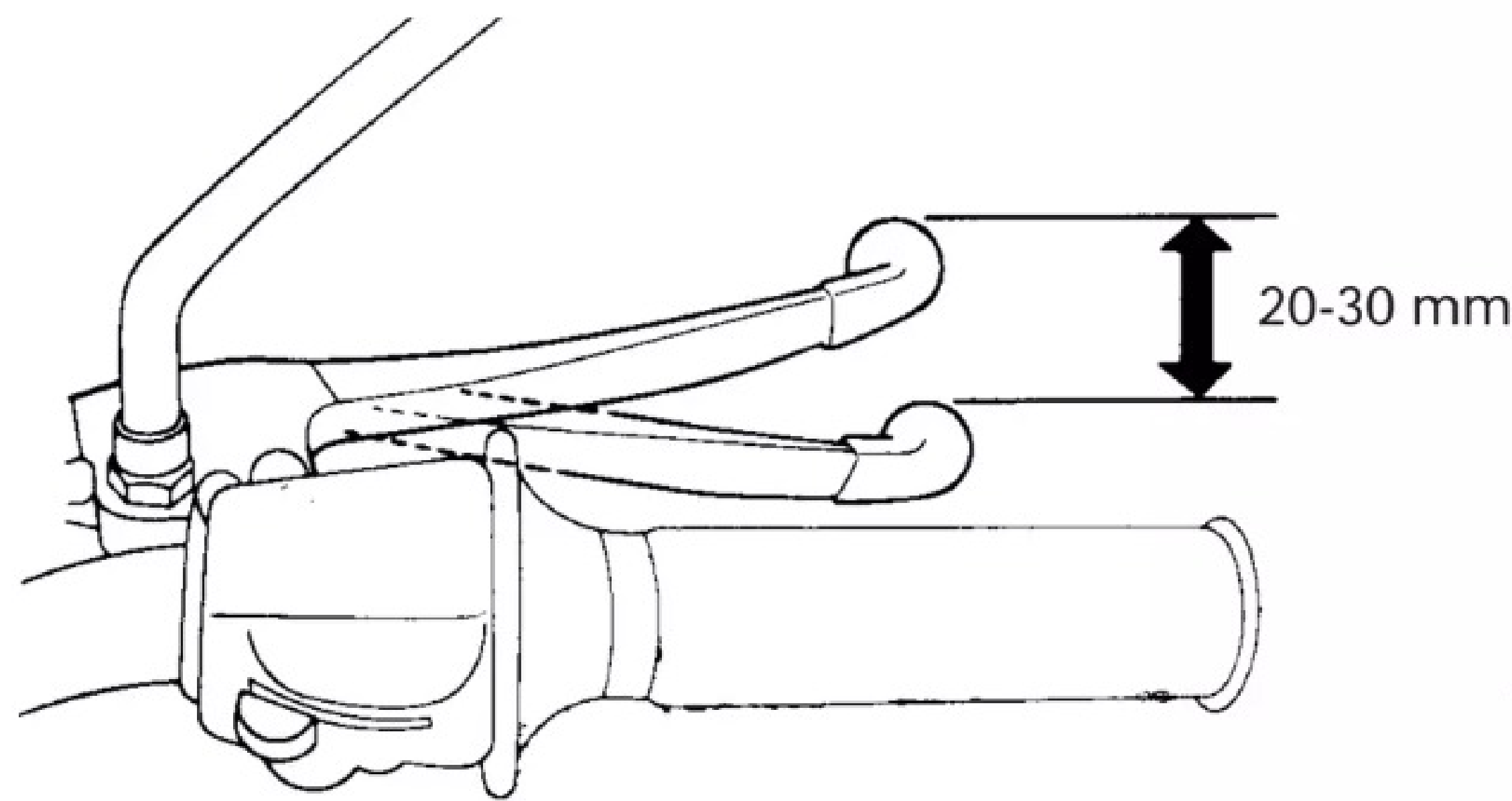
FOLGA MEDIDA NA EXTREMIDADE DA ALAVANCA DO FREIO
