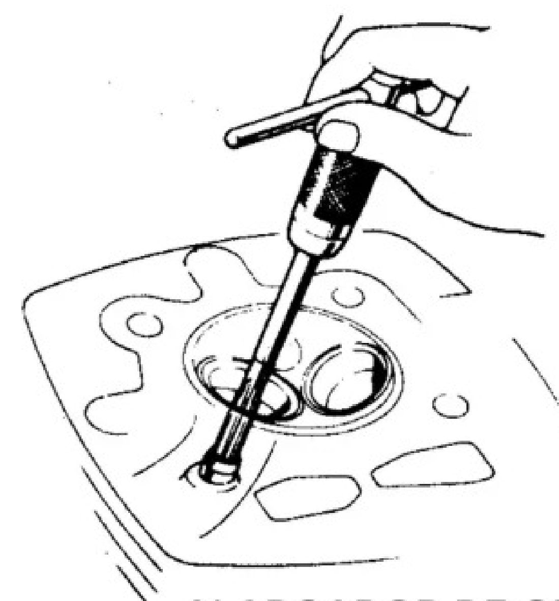
ALARGADOR DE GUIA DE VÁLVULA N.º 07984-0980000
