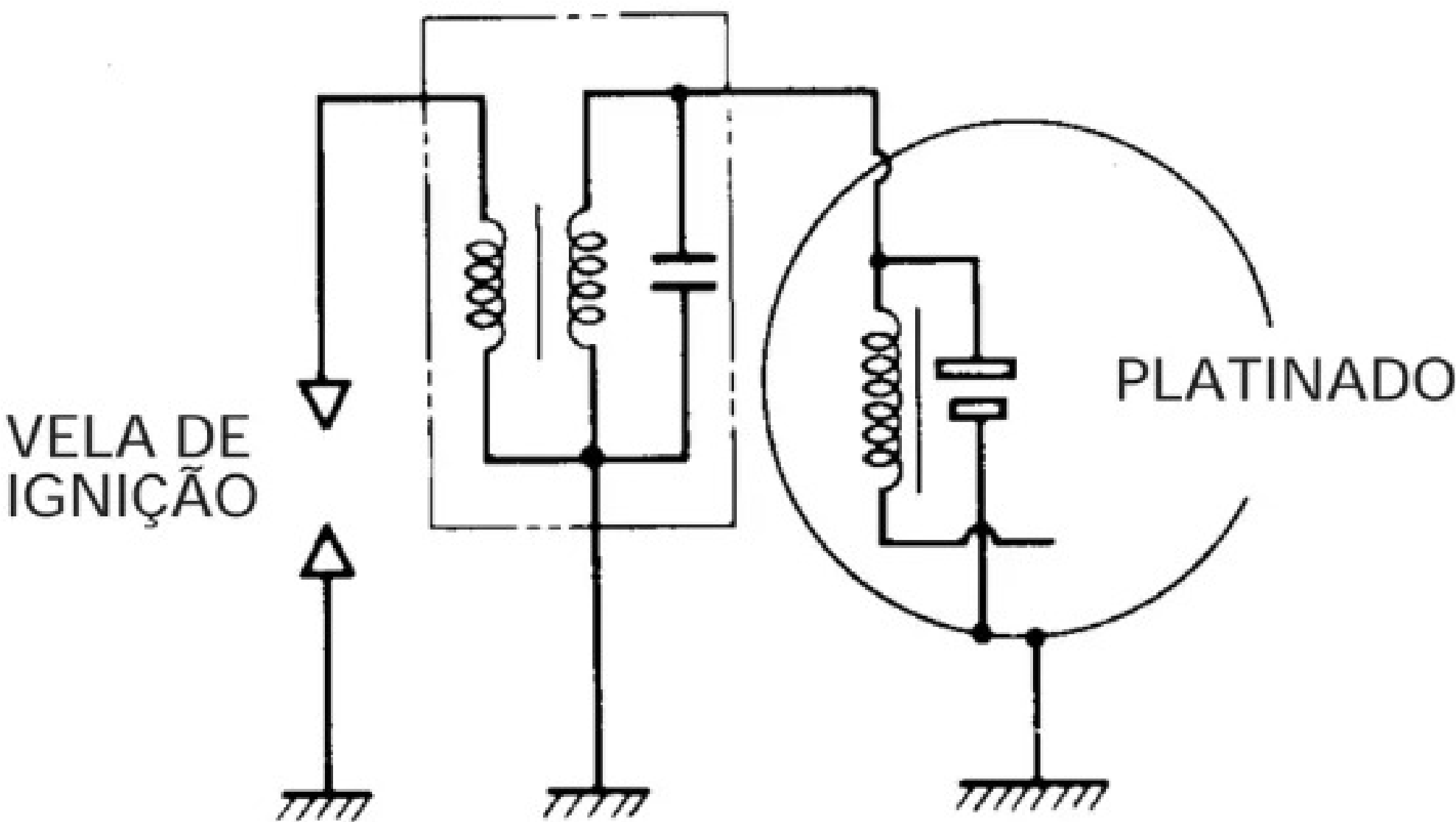
ESQUEMA DO SISTEMA DE IGNIÇÃO BOBINA/CONDENSADOR
