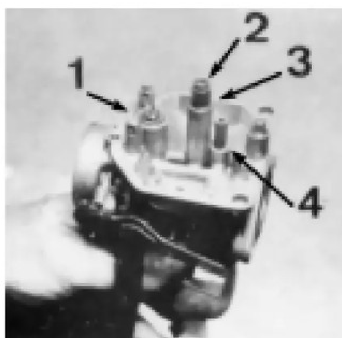
(1) VÁLVULA DA CUBA (2) GICLÊ PRINCIPAL (3) PULVERIZADOR (4) GICLÊ DE MARCHA LENTA
