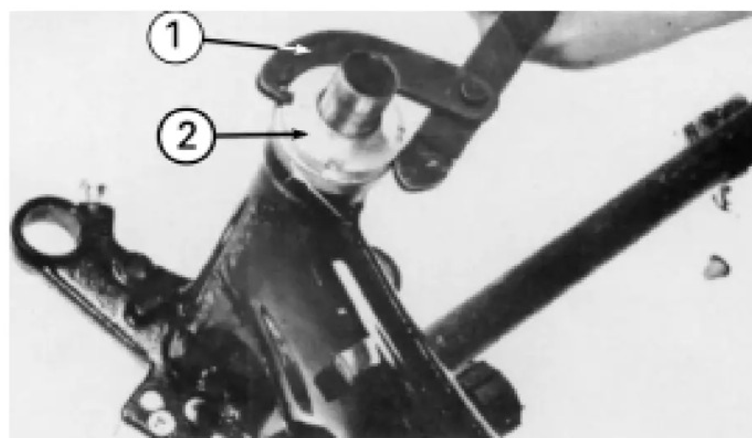
(1) CHAVE ESPECIAL (2) PORCA CILÍNDRICA
