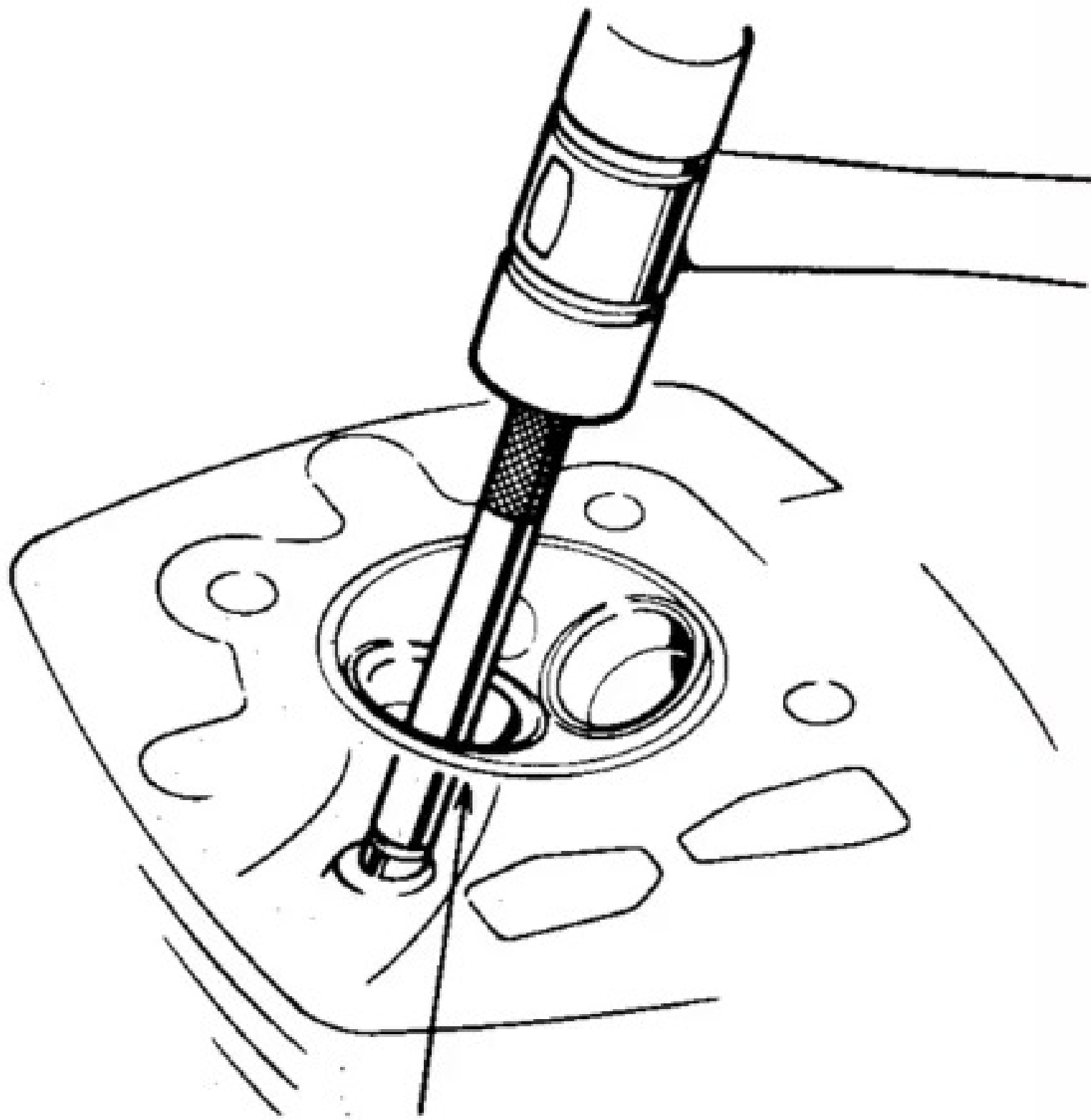
REMOVEDOR DE GUIA DE VÁLVULA (F.E. N.º 07942-3290100)
