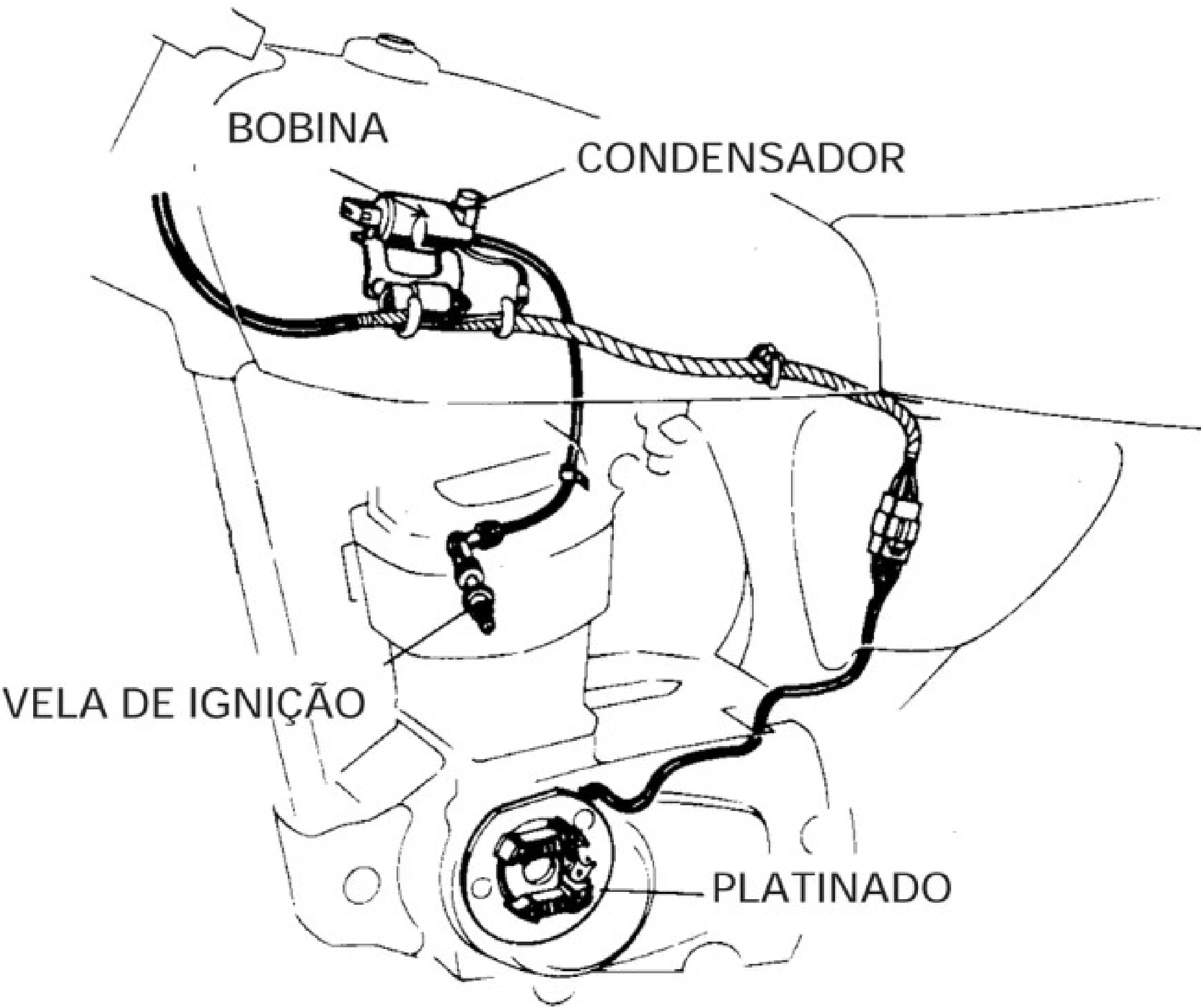
TESTE SIMPLIFICADO DA BOBINA Utilizando apenas lâmpada e bateria)
