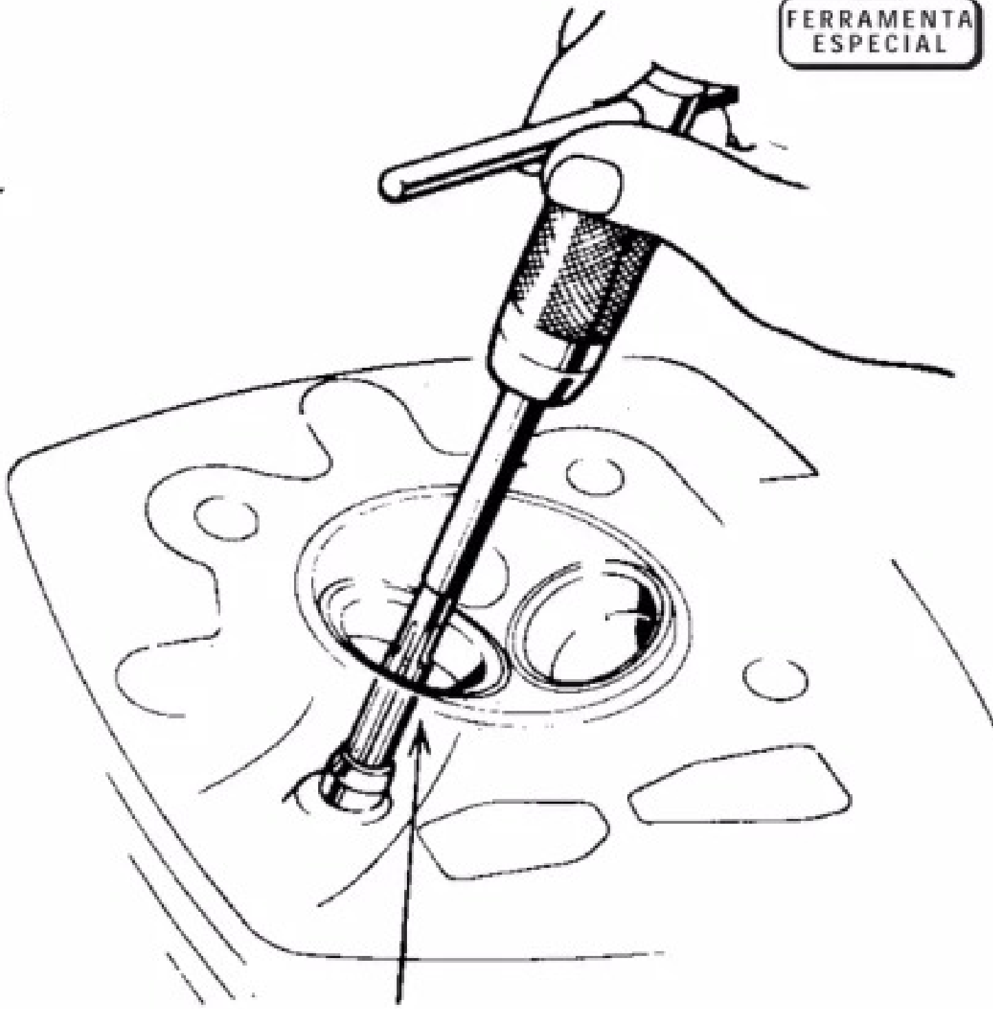
ALARGADOR DE GUIA DE VÁLVULA (F.E. N.º 07984-0980000)
