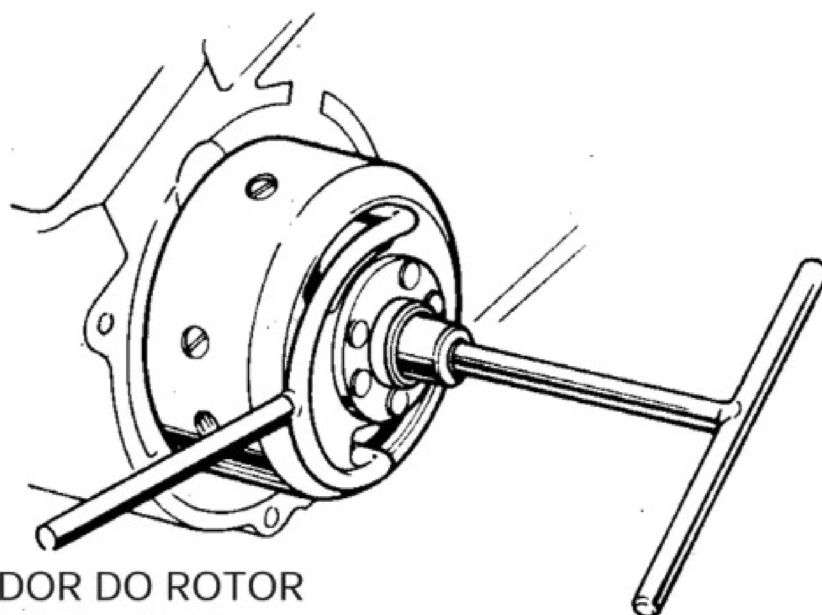
CHAVE ESPECIAL 14 mm N.º 07915-639000
