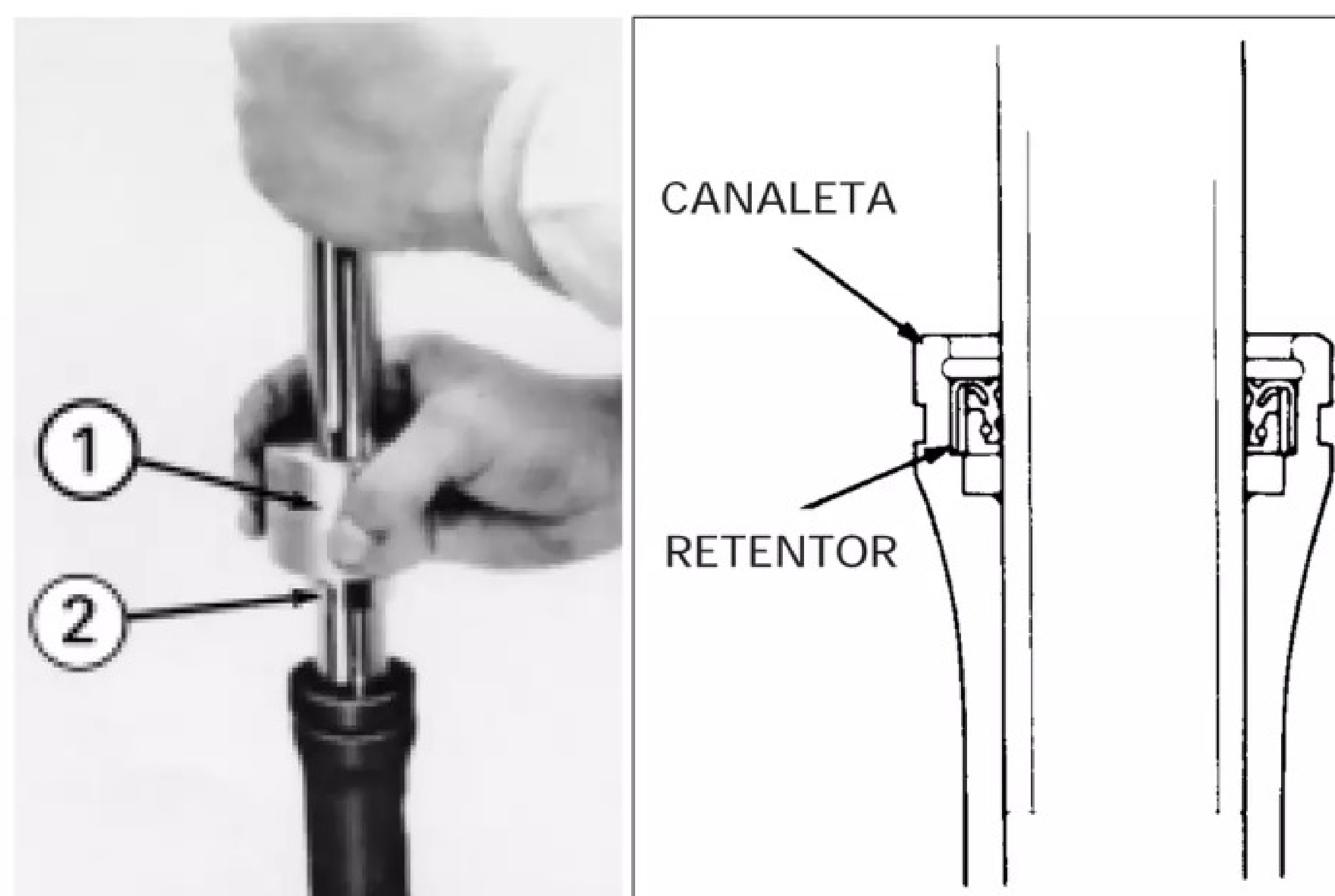
(1) CORPO DA GUIA DO RETENTOR (2) GUIA INTERNA
