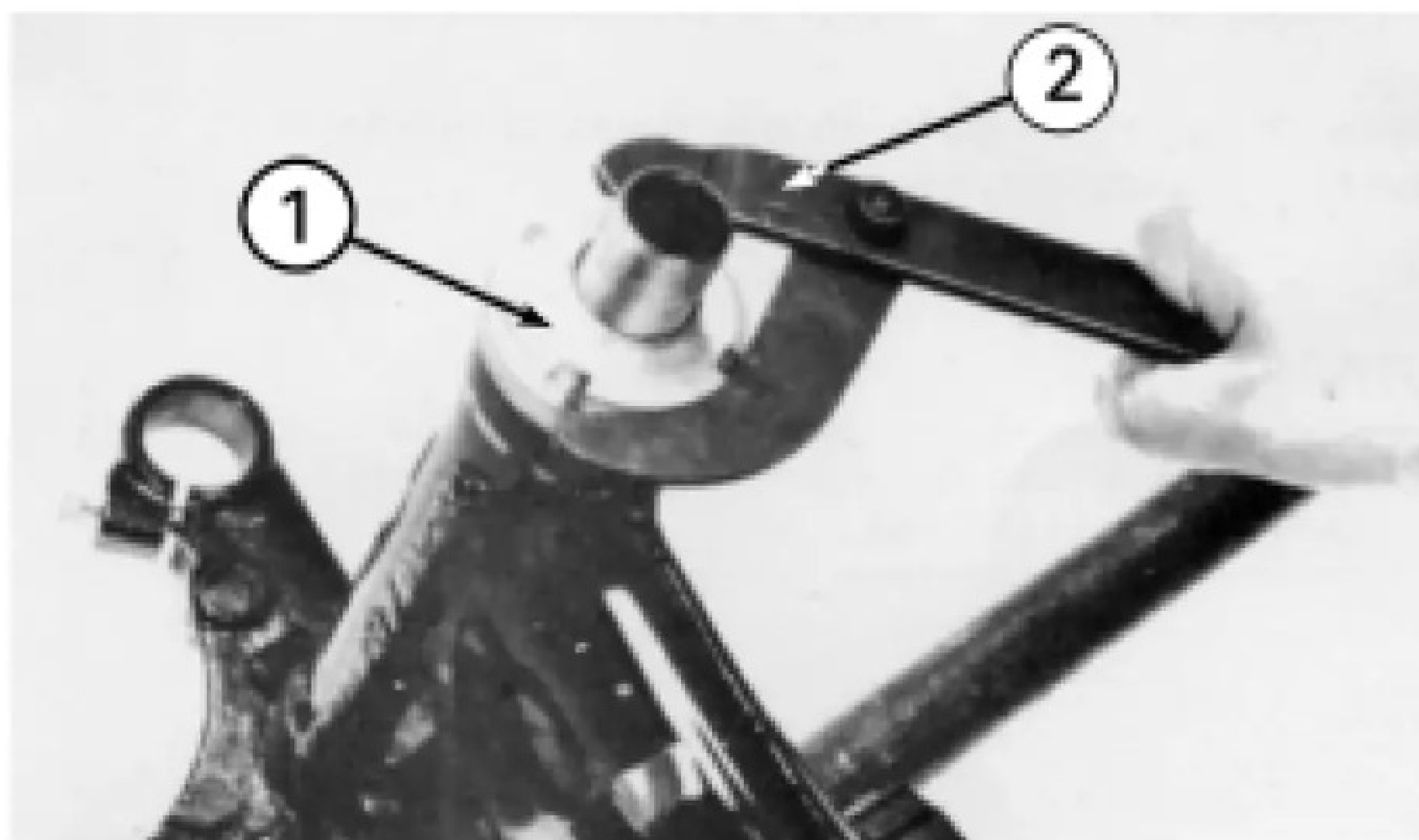
(1) PORCA CILÍNDRICA (2) CHAVE ESPECIAL
