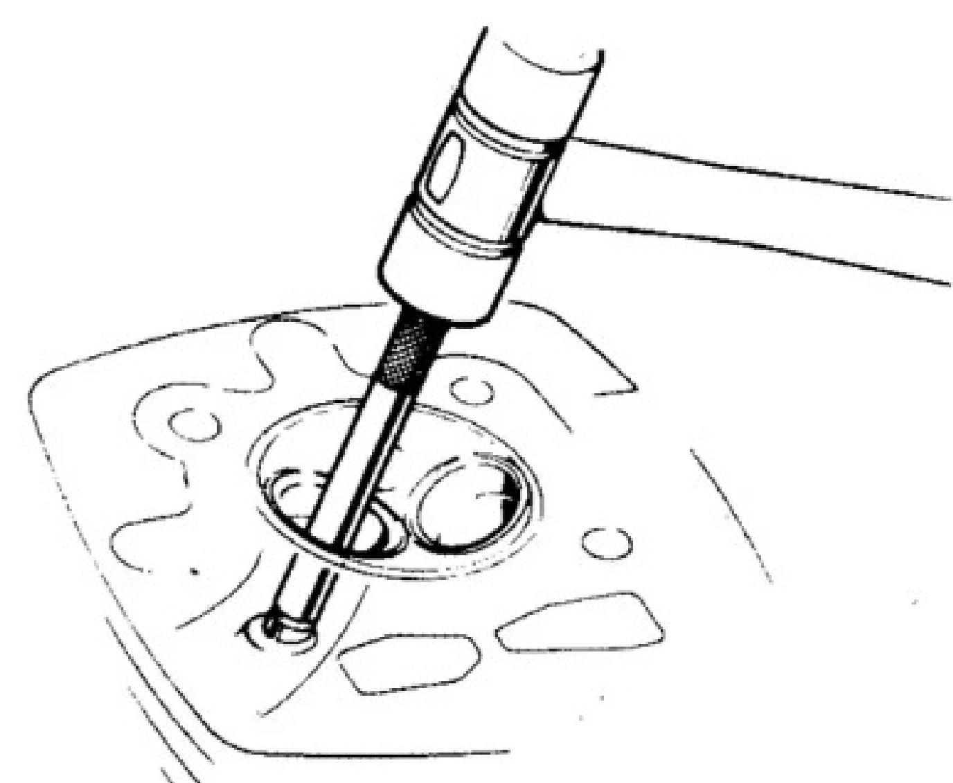
REMOVEDOR DE GUIA DE VÁLVULA N.º 07942-3290100
