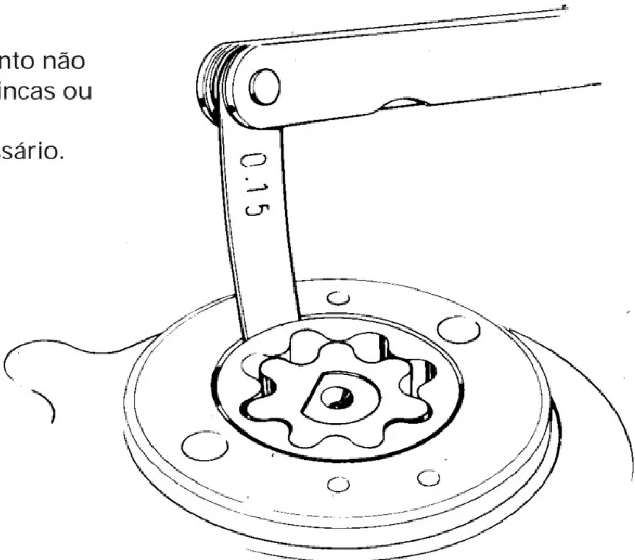
FOLGA ENTRE O ROTOR EXTERNO E A CARÇAÇA
