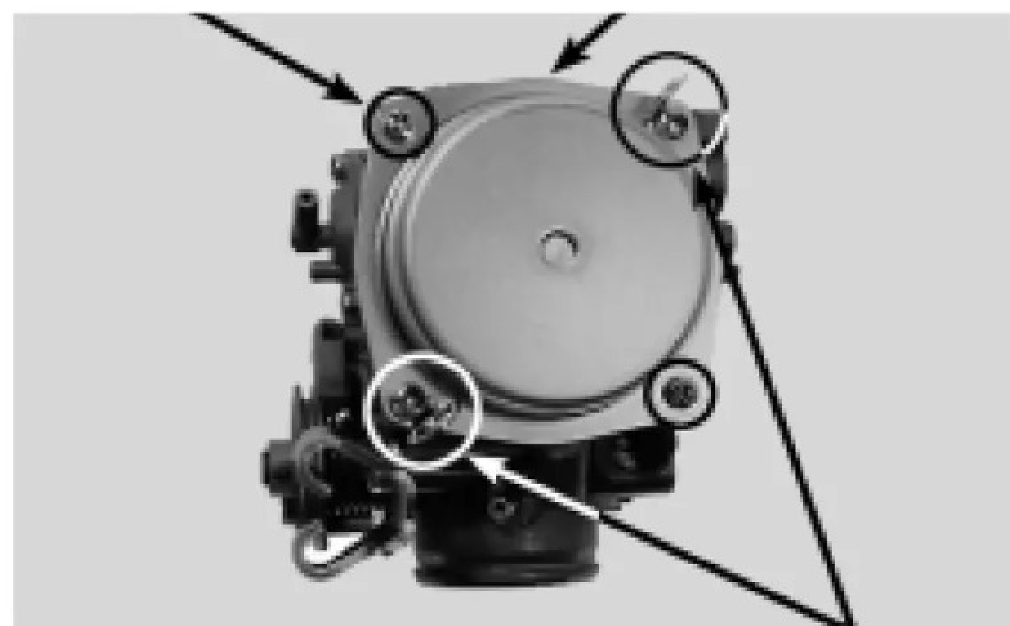
PARAFUSOS/SUPORTES TUBO DE DRENAGEM/TUBO DE RESPIRO
