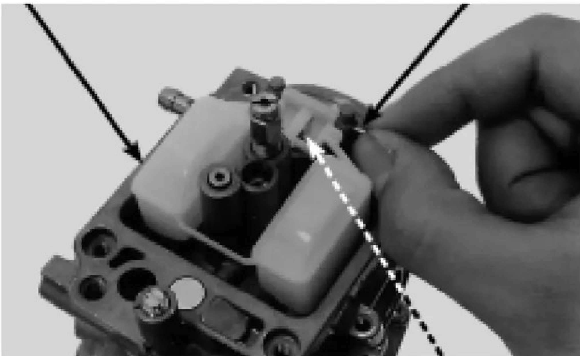
VÁLVULA DA BÓIA
