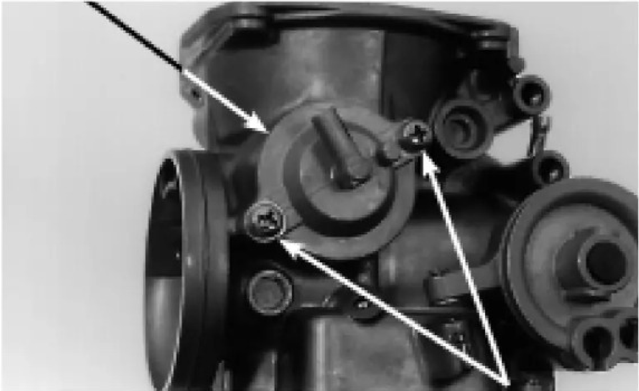
PARAFUSOS DIAFRAGMA/PISTÃO DE VÁCUO
