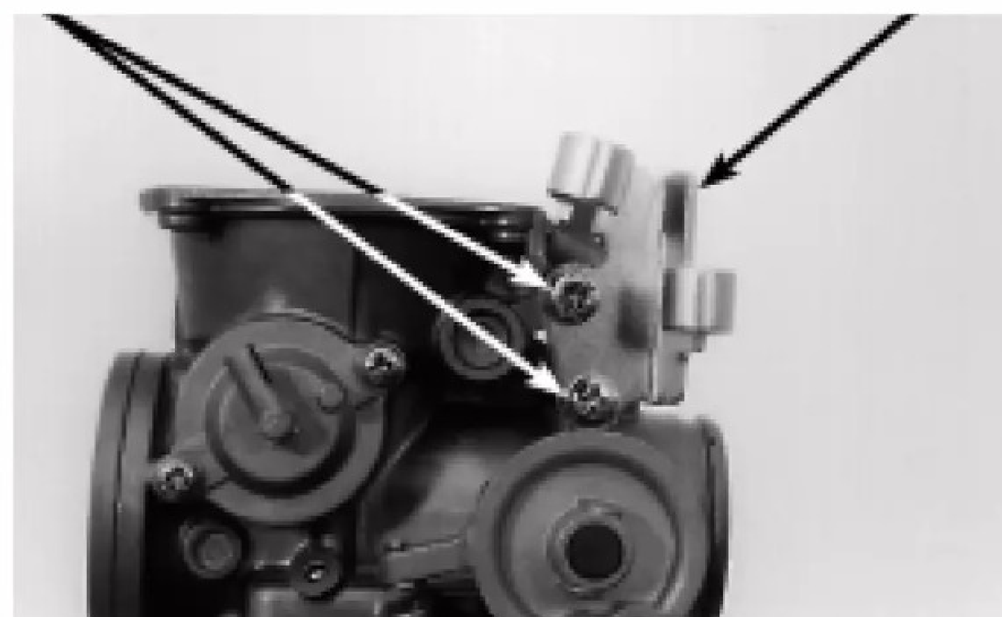
DIAFRAGMA/VÁLVULA DE CORTE DE AR TAMPA PARAFUSOS SUPORTE
