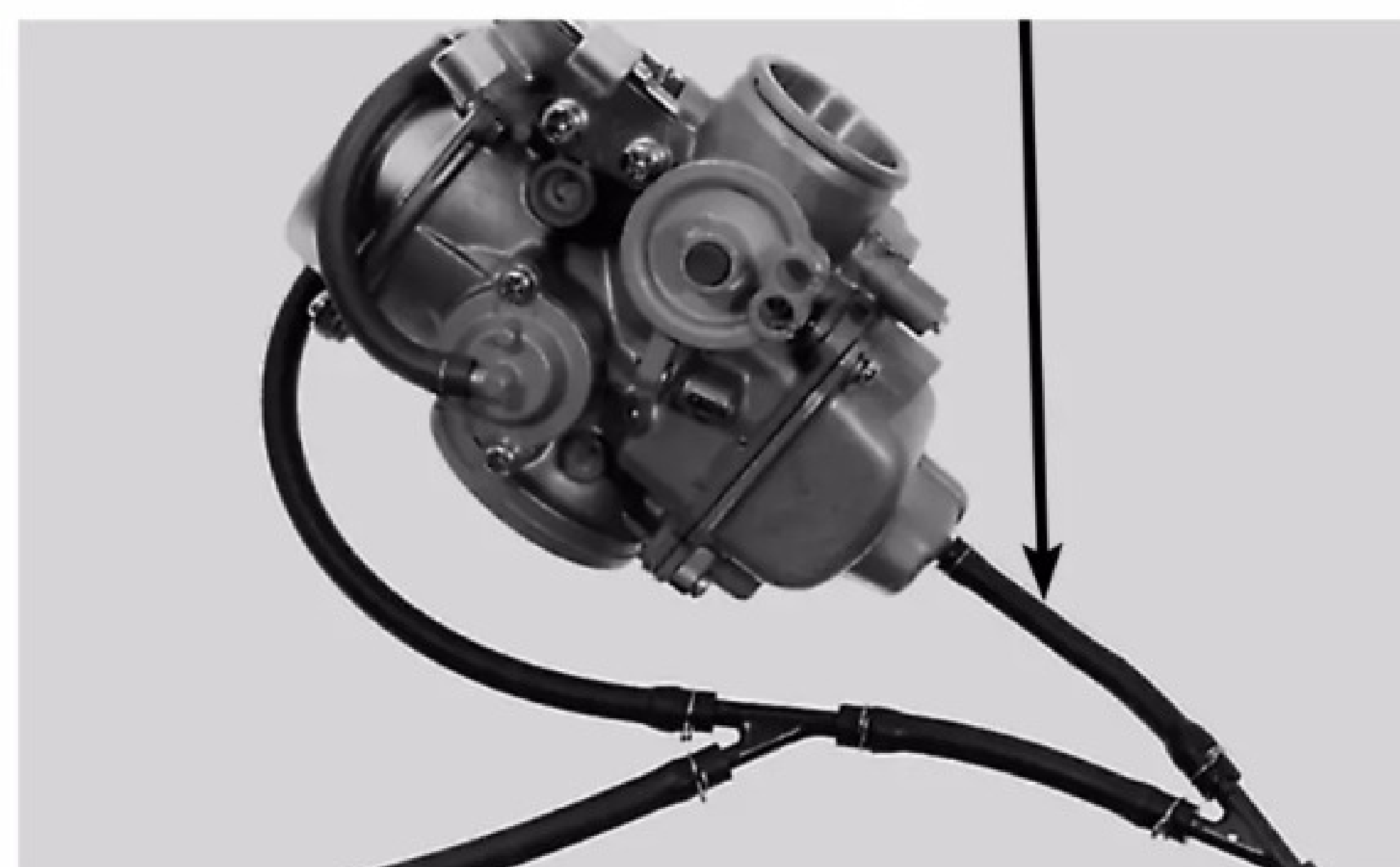
TUBO DE DRENAGEM/TUBO DE RESPIRO
