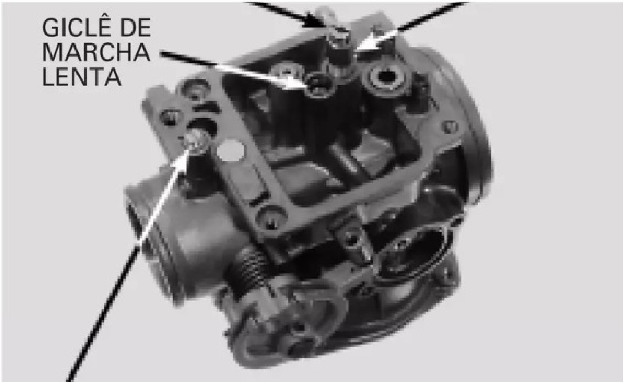
PARAFUSO DE MISTURA
