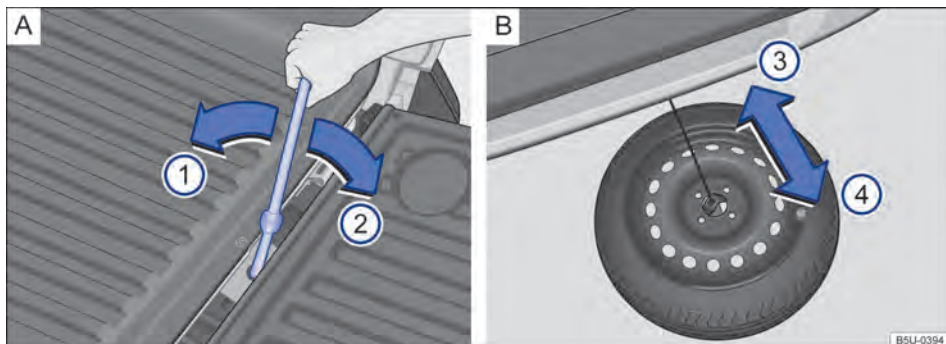
Fig. 192 A) No compartimento de carga: acesso à roda de emergência. B) Sob o veículo: roda de emergência totalmente no piso e retirada de baixo do veículo.
