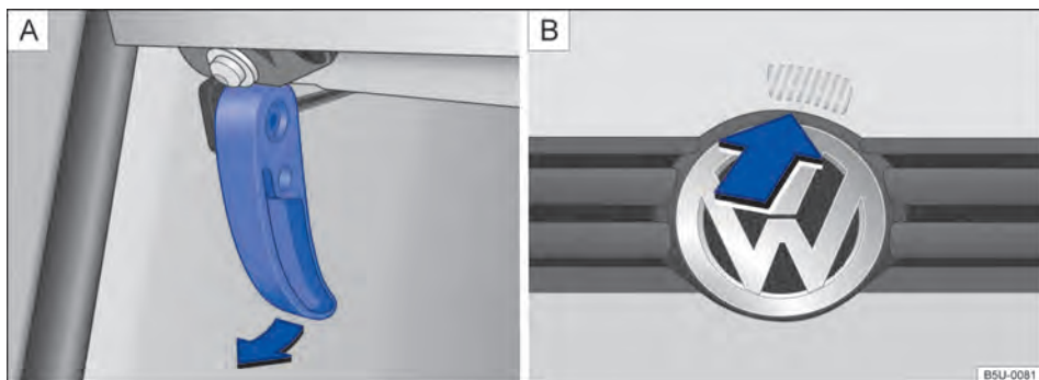
Fig. 178 [A] Alavanca de destravamento da tampa do compartimento do motor na área para os pés do lado do condutor. [B] Alavanca de destravamento na parte interna da tampa do compartimento do motor.
