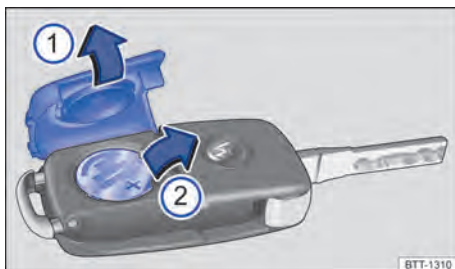
Fig. 54 Chave do veículo com comando remoto: ① Abrir a tampa do alojamento da bateria. ② Remover a bateria.
