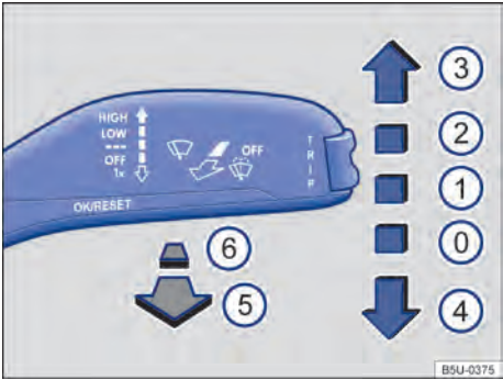
Fig. 83 Comandar os limpadores / lavadores do para-brisa.
