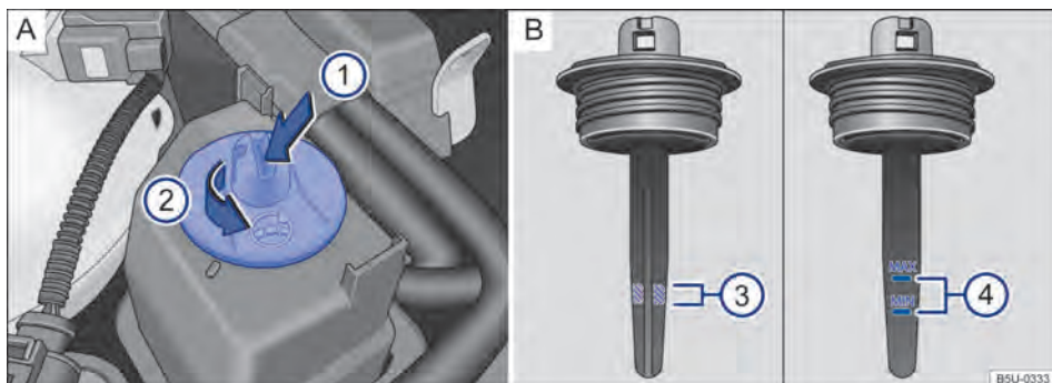
Fig. 104 No compartimento do motor (variante 1): A ) Reservatório do fluido da direção hidráulica. B ) Marcações para controle do nível do fluido da direção hidráulica.
