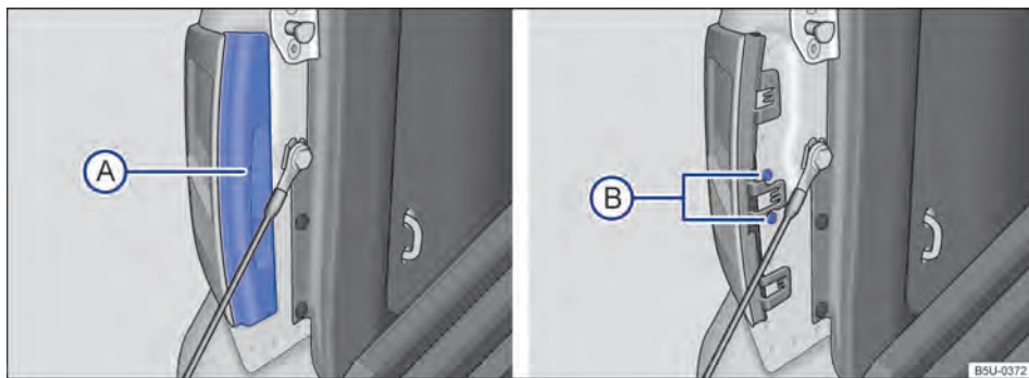
Fig. 164 No compartimento de carga: A desinstalar cobertura, B retirar os parafusos de fixação. ▶
