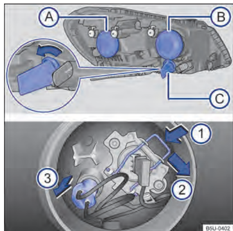
Fig. 159 No compartimento do motor: vista traseira do farol dianteiro com cobertura de borracha (lado esquerdo da ilustração) - (A) farol baixo, (B) farol alto e luz de posição, e (C) indicador de direção. Vista traseira do farol dianteiro sem a cobertura de borracha (lado direito da ilustração): (1) mola de travamento da lâmpada incandescente do farol e (2) luz de posição.
