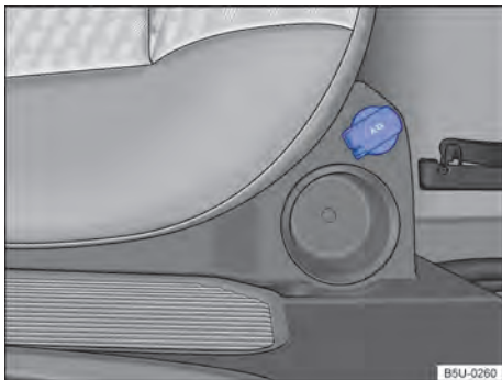
Fig. 138 Na lateral do banco traseiro: tomada 12 V - Nova Saveiro cabine dupla.
