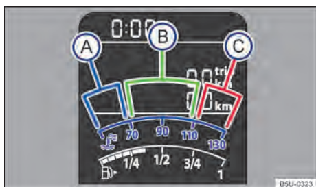
Fig. 20 Indicador de temperatura do líquido de arrefecimento do motor no instrumento combinado (variante 1): (A) área fria; (B) área normal; (C) área de alerta.
