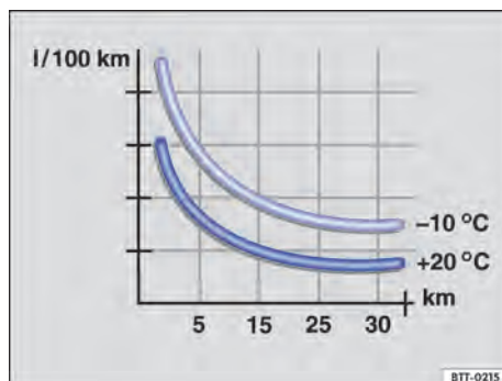
Fig. 100 Consumo de combustível em l/100 km em 2 temperaturas ambiente diferentes.
