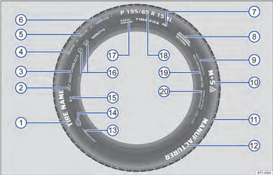
Fig. 194 Inscrição dos pneus internacional (exemplo).
