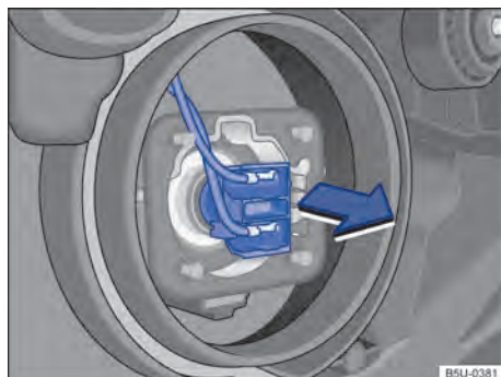
Fig. 160 Acesso à lâmpada incandescente do farol baixo.
