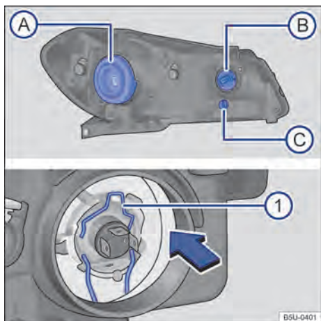
Fig. 157 No compartimento do motor: vista traseira do farol dianteiro com cobertura de borracha (lado esquerdo da ilustração) - (A) farol baixo / alto, (B) indicadores de direção e (C) luz de posição. Vista traseira do farol dianteiro sem a cobertura de borracha (lado direito da ilustração): (1) mola de travamento da lâmpada incandescente do farol baixo / alto.
