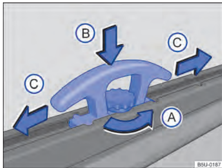
Fig. 143 No compartimento de carga: suporte deslizante para veículos sem capota marítima.
