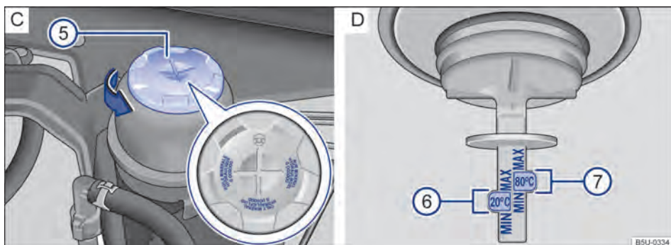
Fig. 105 No compartimento do motor (variante 2): C ) Reservatório do fluido da direção hidráulica. D ) Marcações para controle do nível do fluido da direção hidráulica.
