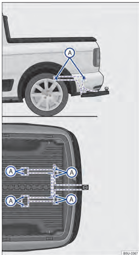
Fig. 149 Pontos de fixação para instalar um dispositivo de reboque posteriormente.
