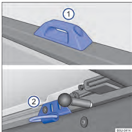
Fig. 142 No compartimento de carga: suportes fixos ① para veículos sem capota marítima e ② para veículos com capota marítima.
