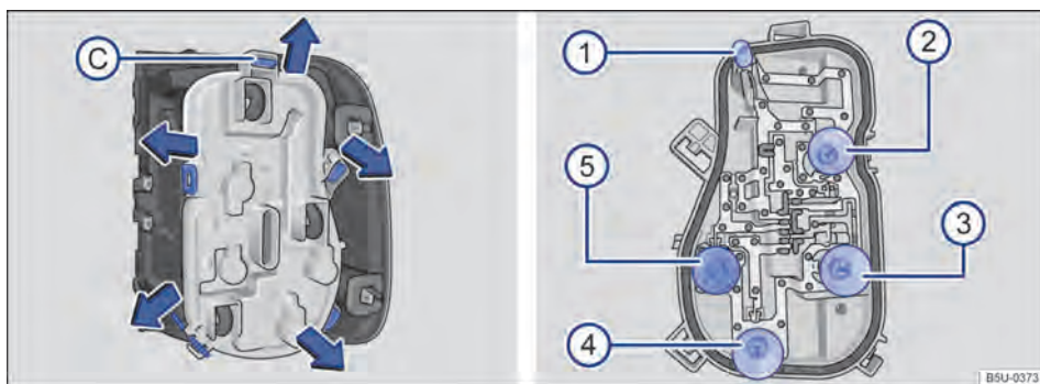
Fig. 165 Lanterna traseira: C desinstalar o suporte das lâmpadas e 1 , 2 , 3 , 4 e 5 desinstalar as lâmpadas.
