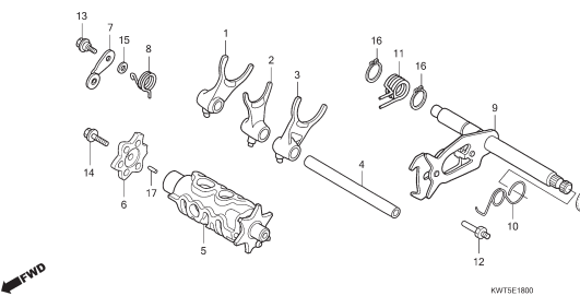
M-18 Tambor Seletor de Marchas
