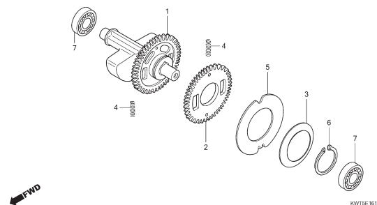
M-16.10 Eixo do Balanceiro
