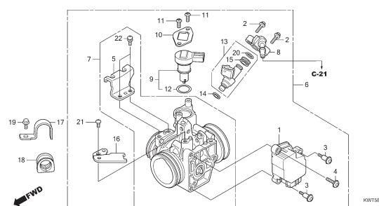
M-22 Corpo do Acelerador
