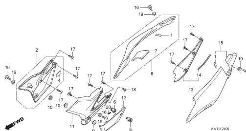
C-24 Tampa Lateral
