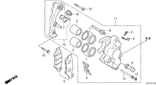
C-12 Cáliber do Freio Dianteiro
