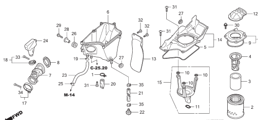
C-25 Filtro de Ar
