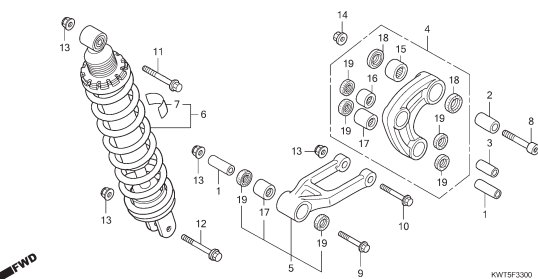
C-33 Amortecedor Traseiro
