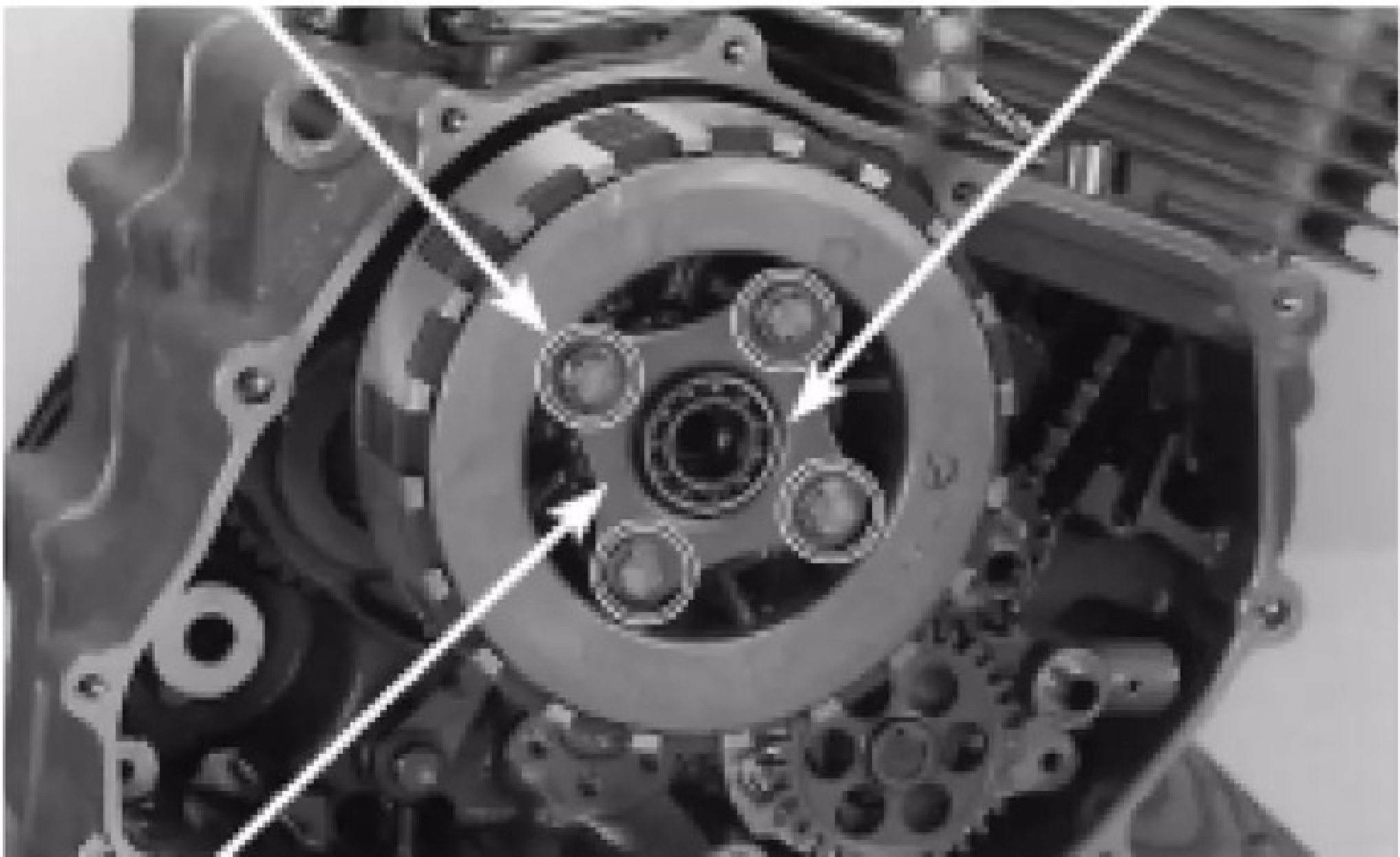
PLACA DE ACIONAMENTO FIXADOR DO CUBO DA EMBREAGEM
