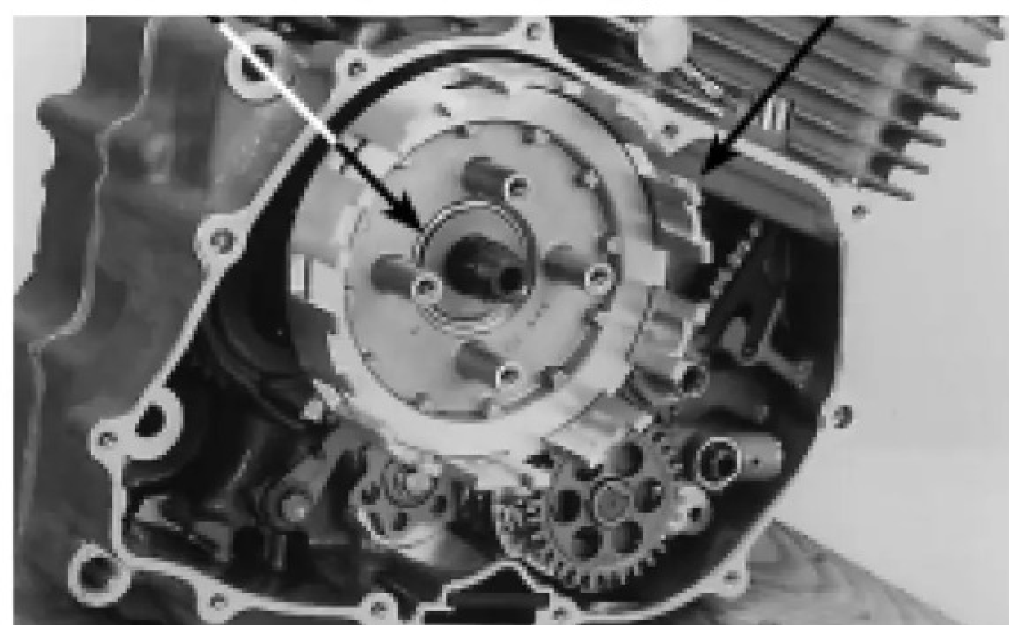
ARRUELA DE ENCOSTO CARCAÇA DA EMBREAGEM
