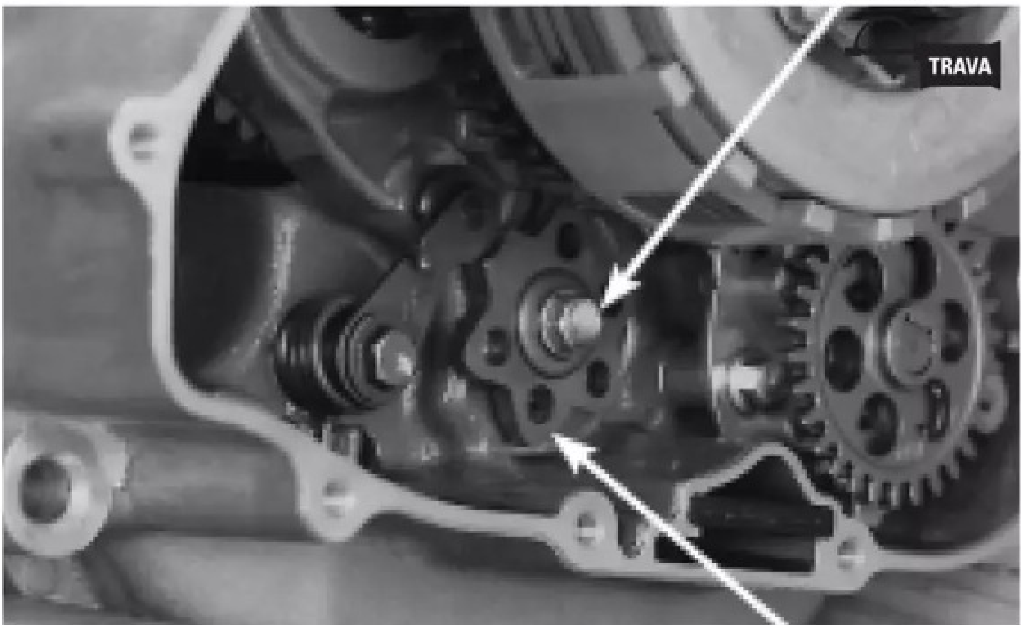
EXCÊNTRICO POSICIONADOR DE MARCHAS RETENTOR DE PÓ
