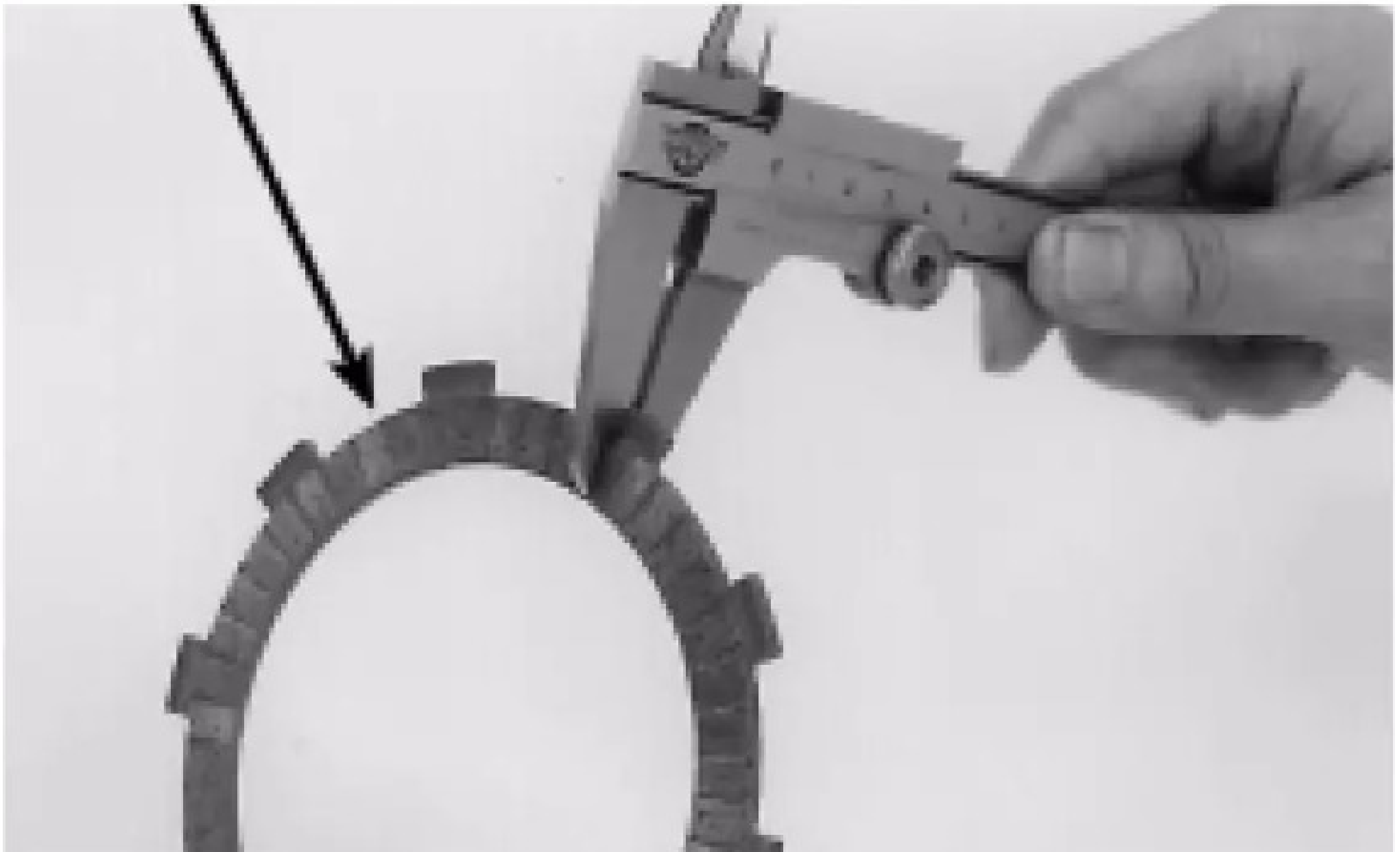
DISCO DA EMBREAGEM
