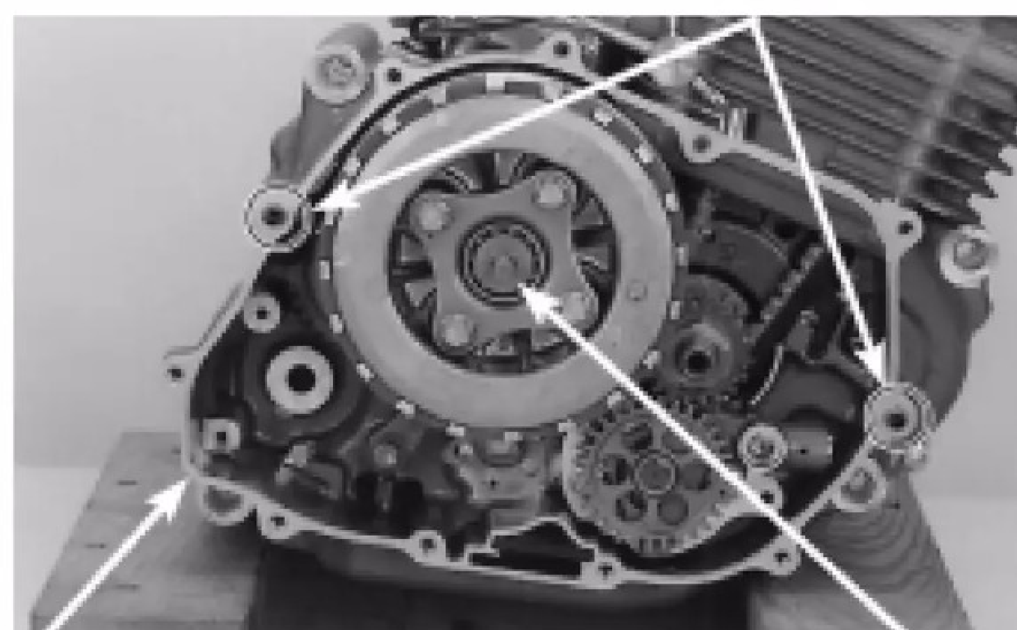
JUNTA HASTE DE ACIONAMENTO
