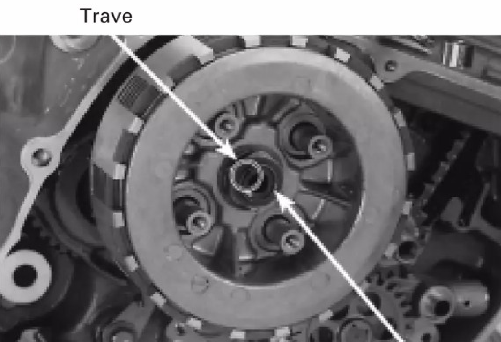
Trave PORCA-TRAVA
