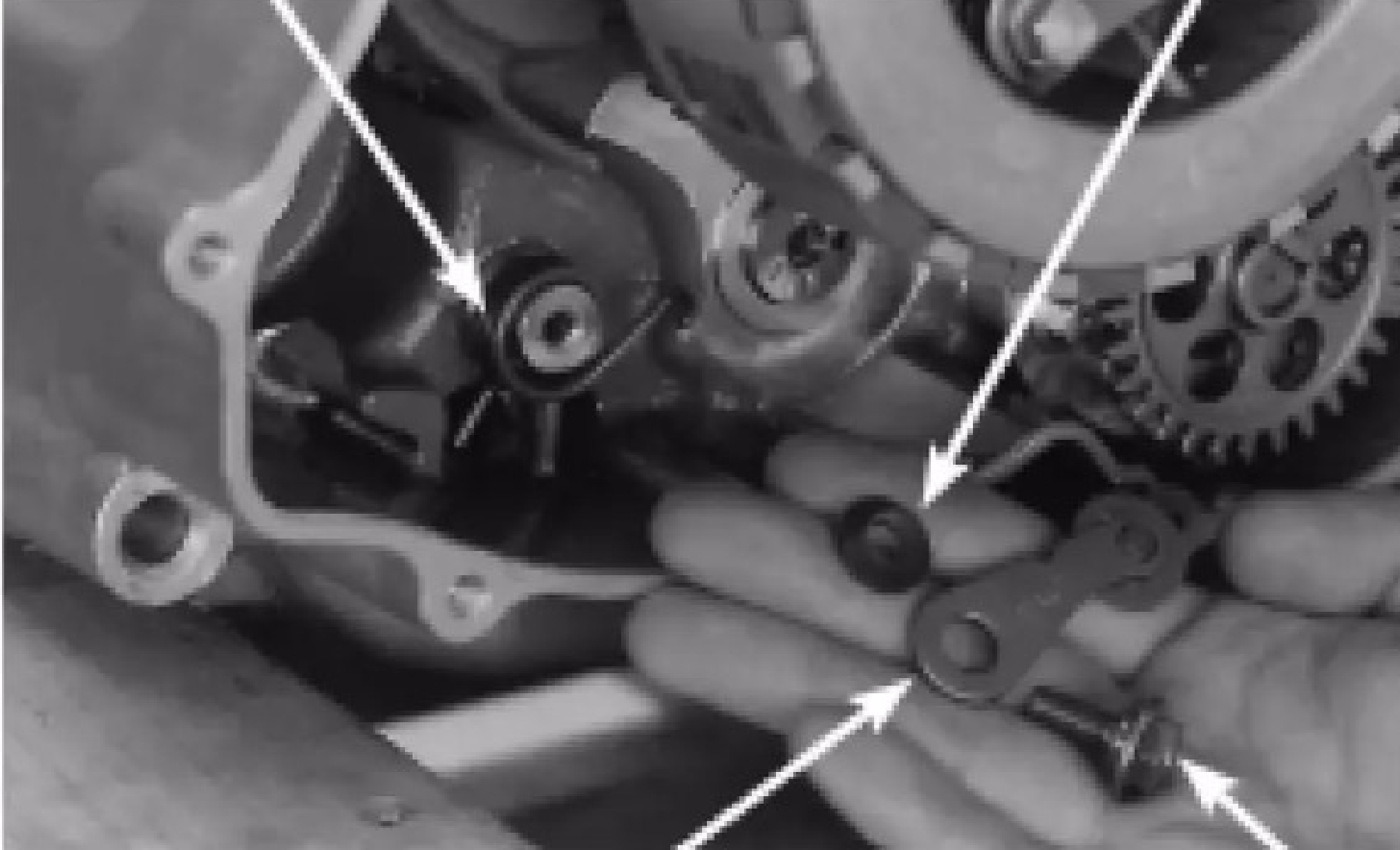
POSICIONADOR DE MARCHAS PARAFUSO
