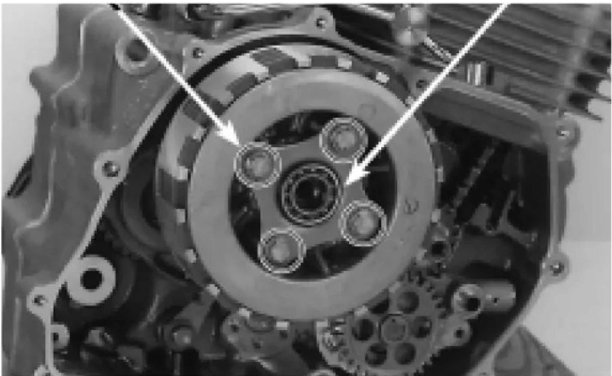
PARAFUSO/MOLA
