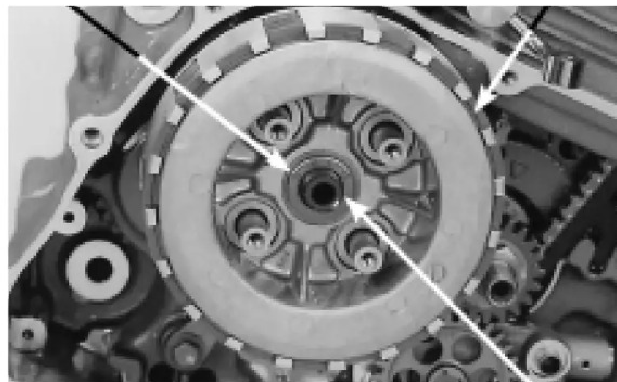
ARRUELA CÔNICA
