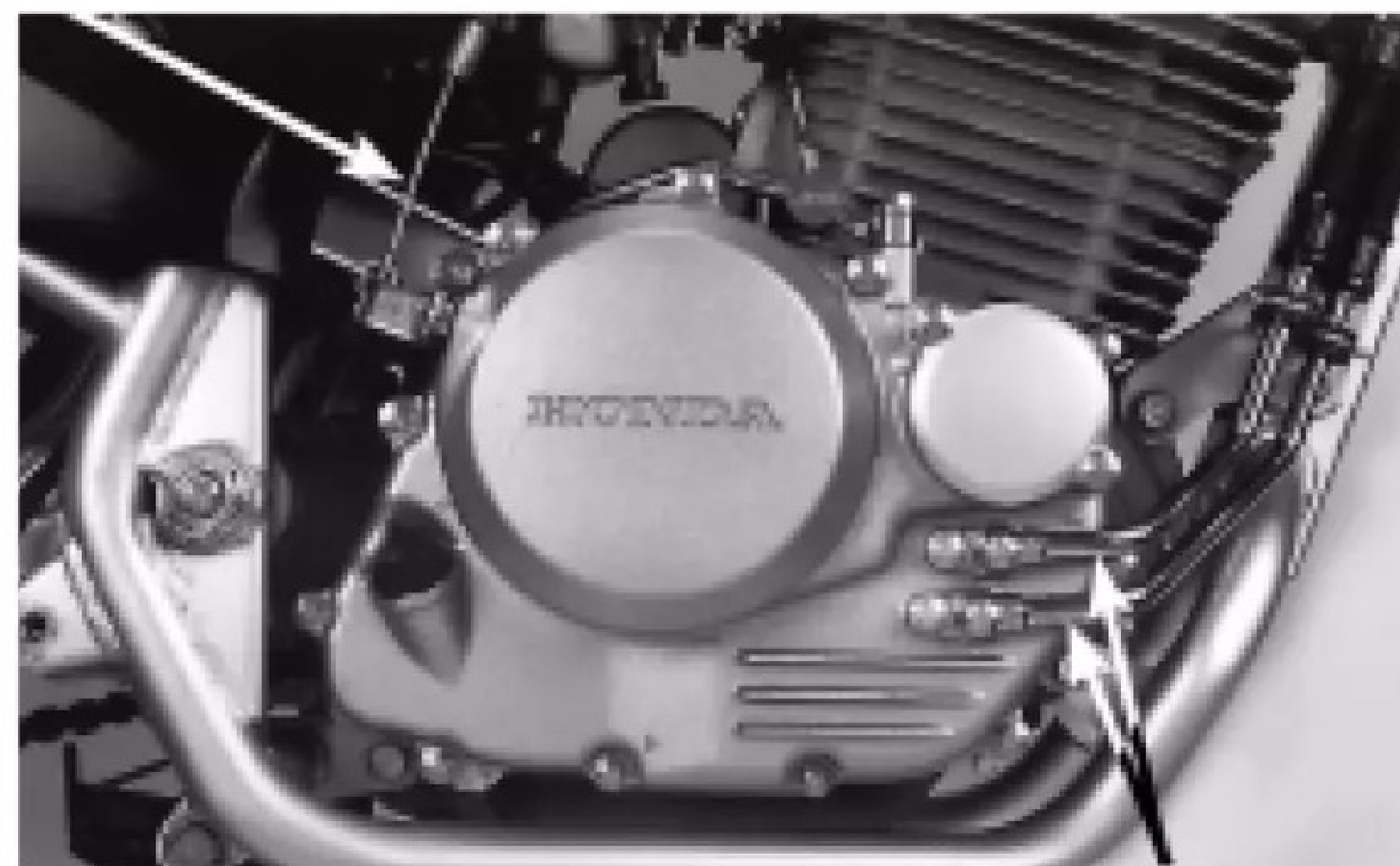
TUBOS DE ÓLEO DO RADIADOR PARAFUSO PARAFUSO ARRUELAS DE VEDAÇÃO
