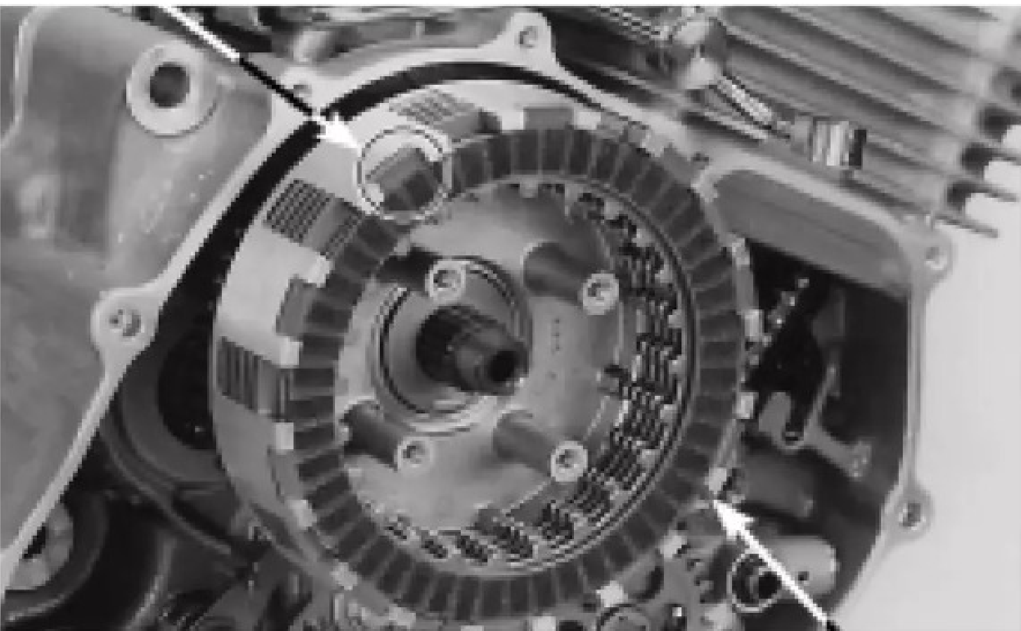
DISCO DE EMBREAGEM EXTERNO ARRUELA MARCA "OUT SIDE" CUBO DA EMBREAGEM
